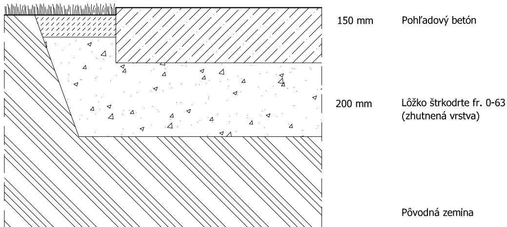
REZ 1-1 VZOROVÝ REZ BETÓNOVOU SPEVNENOU PLOCHOU
