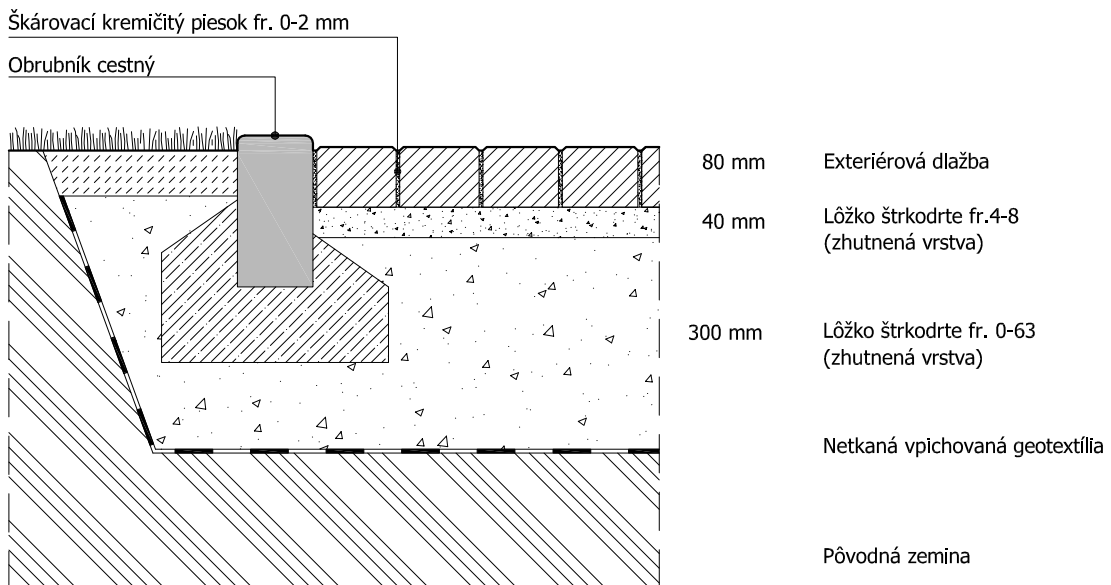
REZ 2-2 VZOROVÝ REZ EXTERIÉROVOU DLAŽBOU ULOŽENOU DO ŠTRKOVÉHO LÔŽKA
